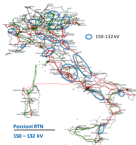
Figura 11 - Aree a maggiore criticità per la sicurezza sulla rete secondaria
