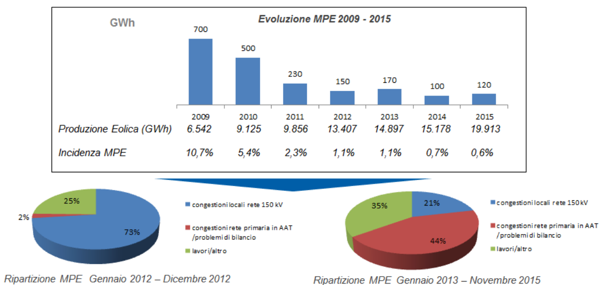
Figura 21 - Mancata Produzione Eolica (MPE) Gennaio-Novembre 2015 – dati provvisori impianti connessi rete AT
