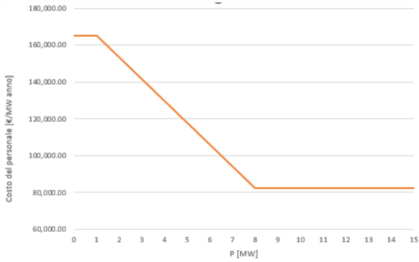
Figura 3-1 Andamento del costo del personale in funzione della taglia
