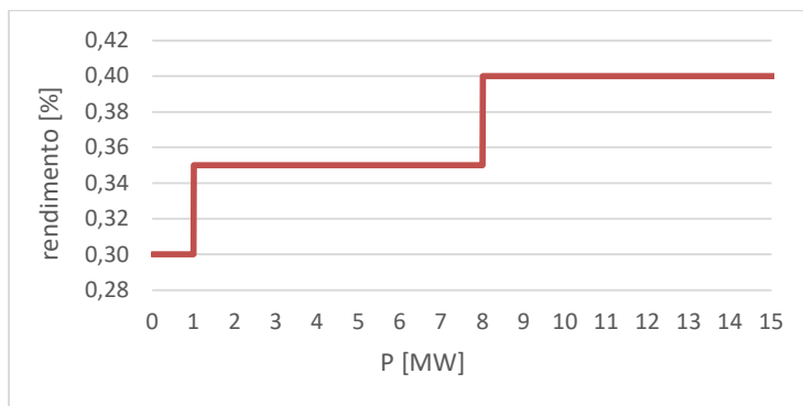
Figura 2-1 Rendimento in funzione della potenza
