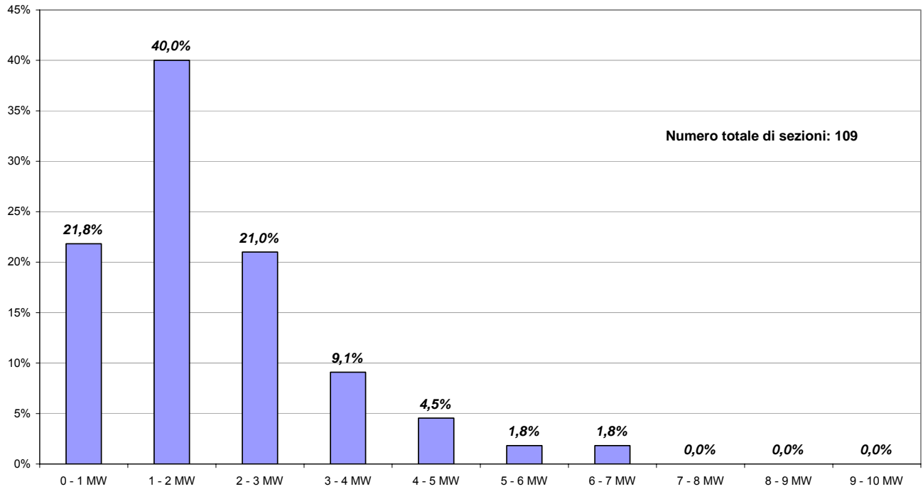
Figura 4.26: Distribuzione delle sezioni con turbine a vapore in contropressione per la produzione combinata di energia elettrica e calore tra le varie classi di potenza nell'ambito della GD.
