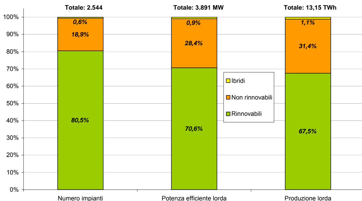
Figura 4.2: Impianti alimentati da fonti rinnovabili, non rinnovabili e impianti ibridi nella GD.
