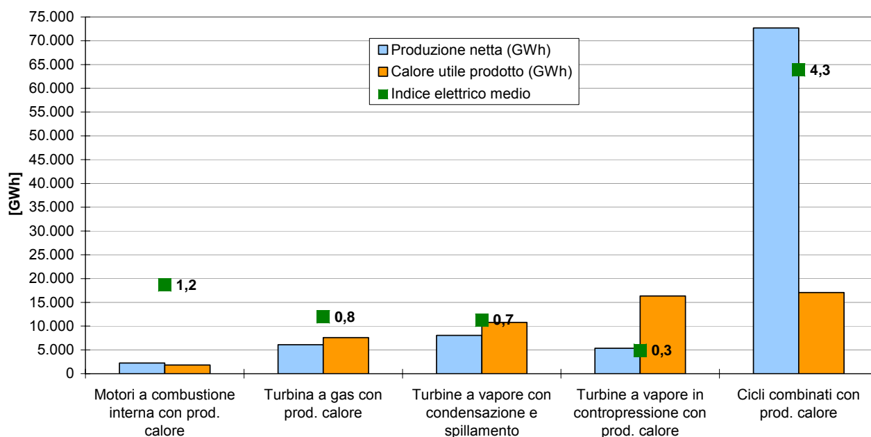
Figura 4.32: Indici elettrici medi per le diverse tecnologie utilizzate per la produzione combinata di energia elettrica e calore nell'ambito del parco termoelettrico complessivo italiano.
