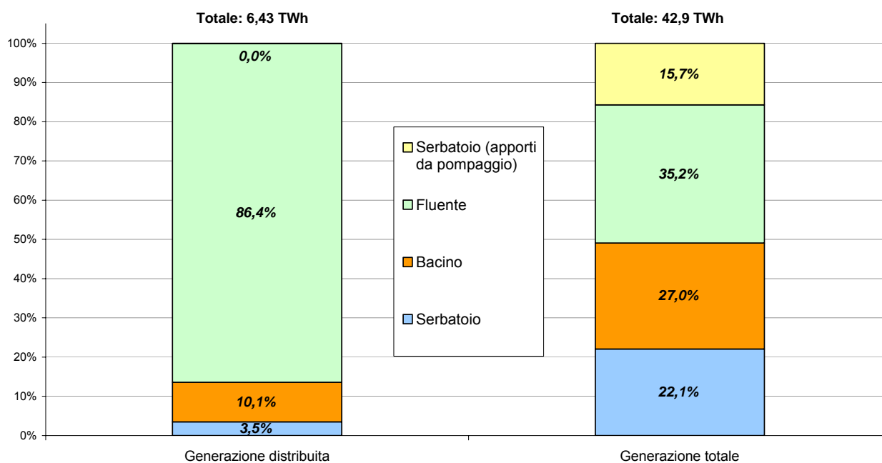
Figura 4.13: Energia elettrica prodotta da impianti idroelettrici nella GD e nella generazione totale.
