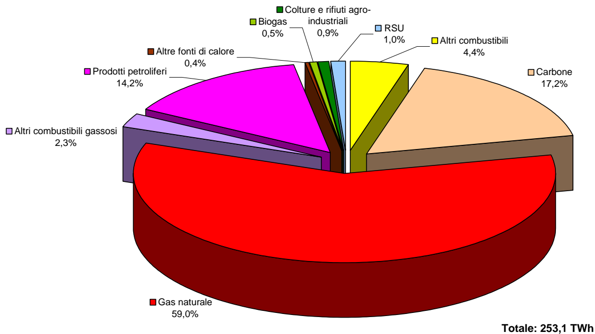
Figura 7: Produzione di energia elettrica dalle diverse fonti utilizzate nell'ambito della generazione termoelettrica nazionale totale nel 2005.
