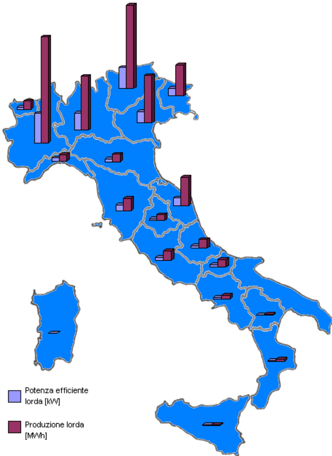
Figura 4.41: Dislocazione regionale degli impianti idroelettrici di PG (Potenza efficiente lorda totale: 421 MW; Produzione lorda totale: 1.472 GWh).
