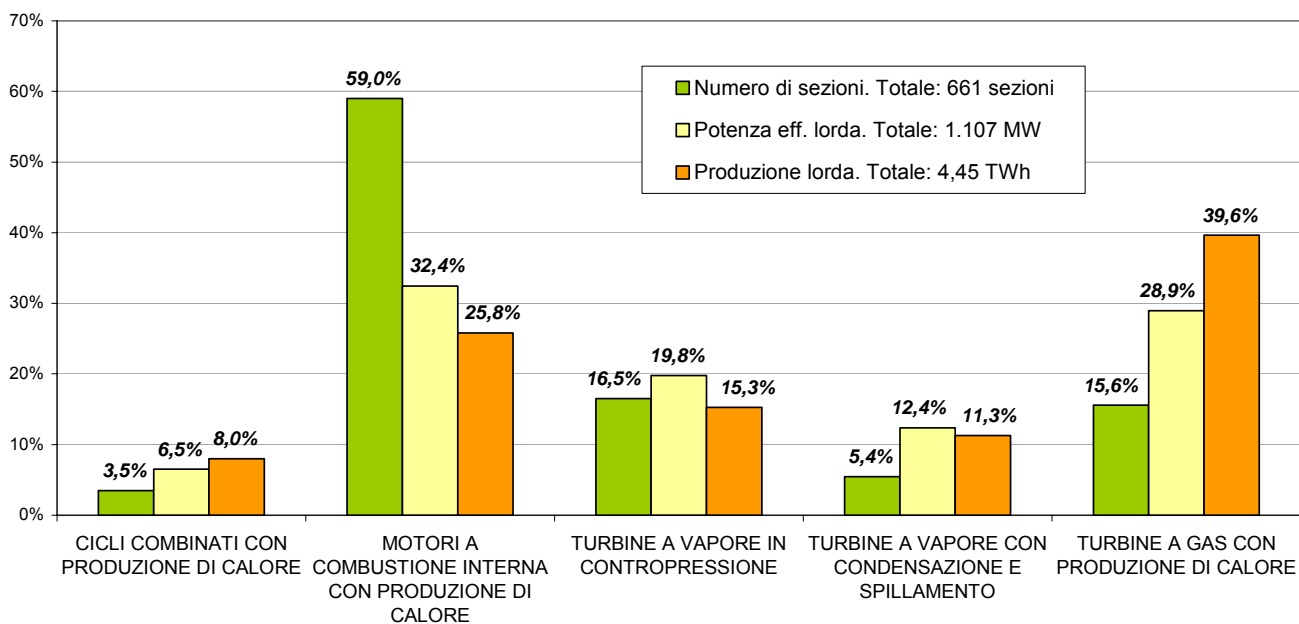
Figura 4.29: Ripartizione delle sezioni degli impianti termoelettrici tra le diverse tecnologie utilizzate per la produzione combinata di energia elettrica e calore nell'ambito della GD.
