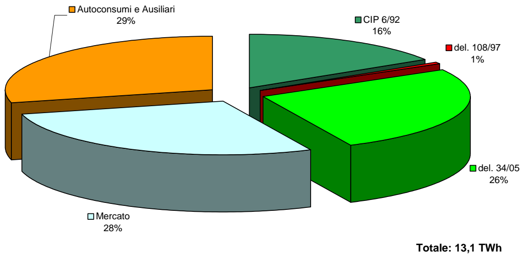
Figura 3: Ripartizione dell'energia elettrica prodotta nell'ambito della GD fra mercato, autoconsumi e regimi di ritiro amministrato.
