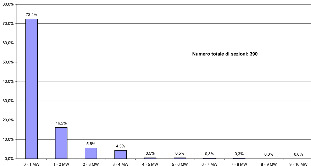
Figura 4.25: Distribuzione delle sezioni con motori a combustione interna per la produzione combinata di energia elettrica e calore tra le varie classi di potenza nell'ambito della GD.
