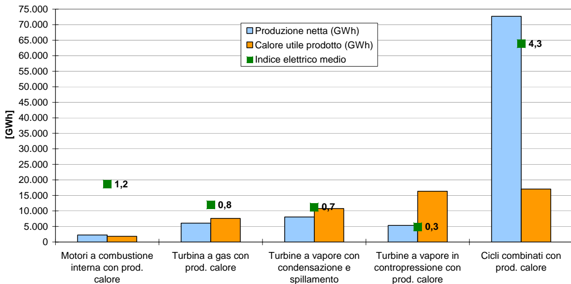
Figura 11: Indici elettrici medi per le diverse tecnologie utilizzate per la produzione combinata di energia elettrica e calore relativi al parco di generazione nazionale nel 2005.
