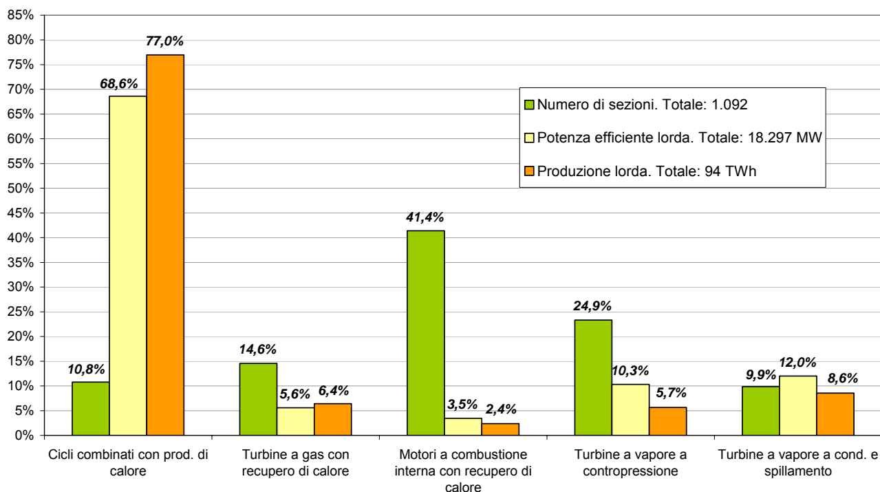
Figura 4.30: Ripartizione delle sezioni degli impianti termoelettrici tra le diverse tecnologie utilizzate per la produzione combinata di energia elettrica e calore nell'ambito del parco termoelettrico complessivo italiano.
