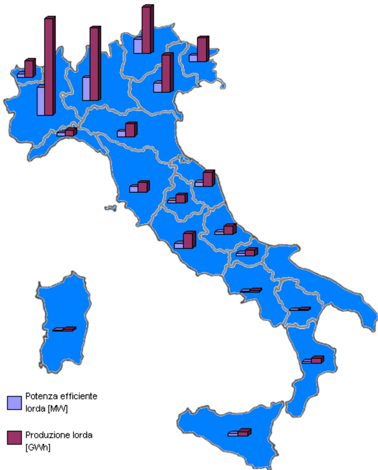
Figura 4.15: Dislocazione regionale degli impianti idroelettrici di GD (Potenza efficiente lorda totale: 2.008 MW; Produzione lorda totale: 6.428 GWh).
