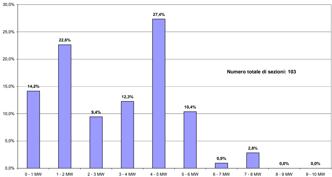
Figura 4.27: Distribuzione delle sezioni con turbine a gas per la produzione combinata di energia elettrica e calore tra le varie classi di potenza nell'ambito della GD.
