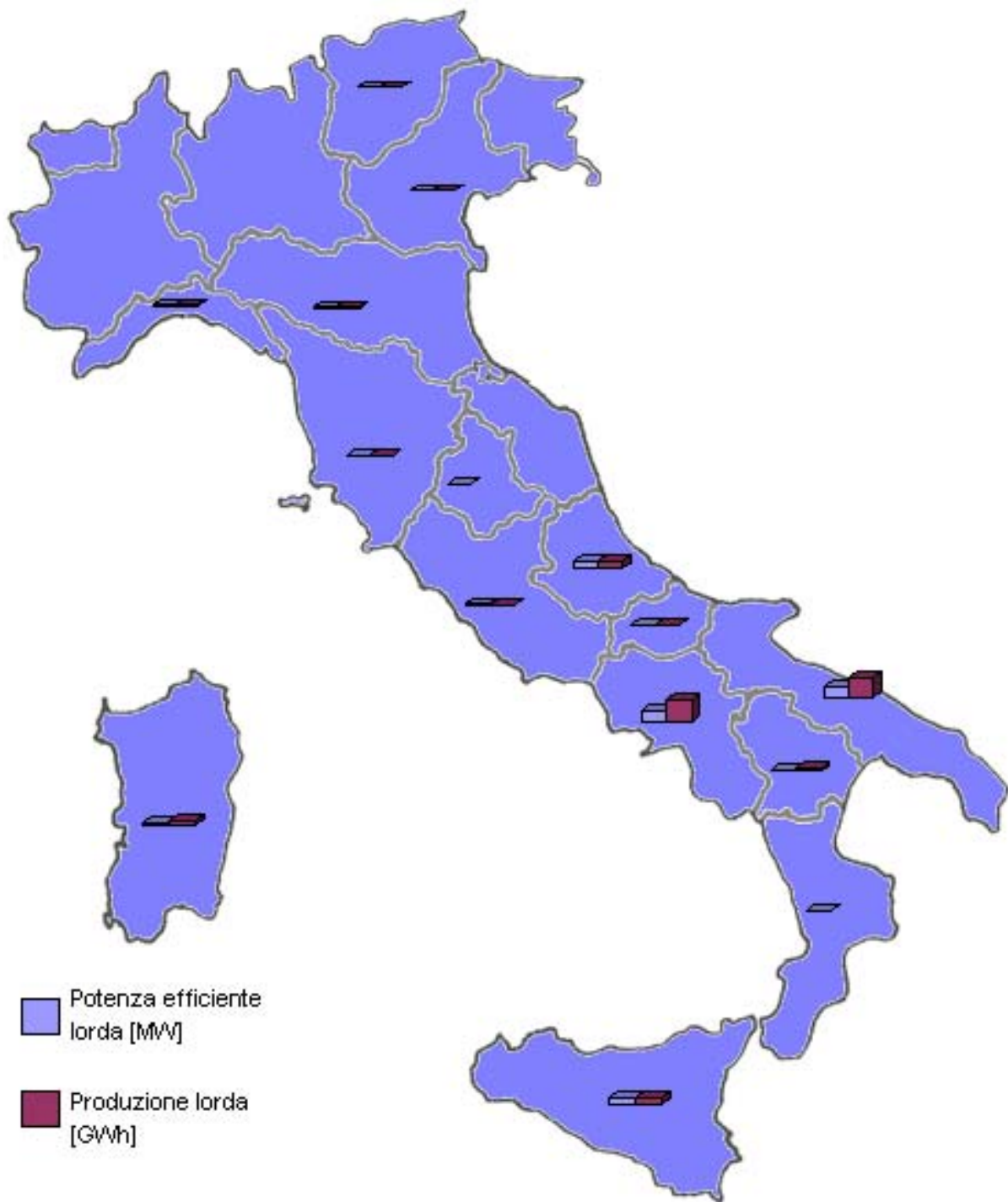
Figura 4.16: Dislocazione regionale degli impianti eolici di GD (Potenza efficiente lorda totale: 269 MW; Produzione lorda totale: 401 GWh).
