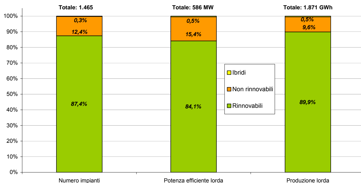
Figura 4.34: Impianti da fonti rinnovabili, non rinnovabili e impianti ibridi nella PG.
