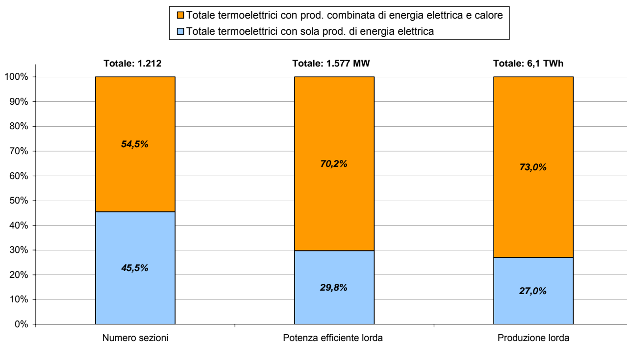
Figura 4.5: Impianti termoelettrici nell’ambito della GD.
