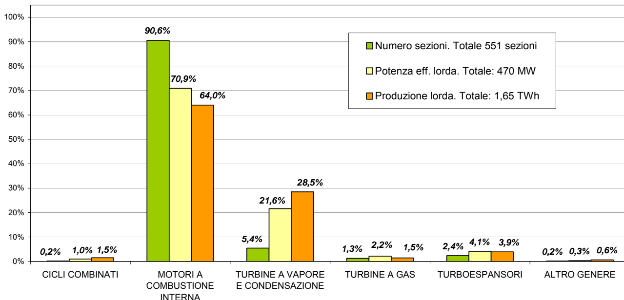
Figura 4.28: Ripartizione delle sezioni degli impianti termoelettrici tra le diverse tecnologie utilizzate per la sola produzione di energia elettrica nell'ambito della GD.
