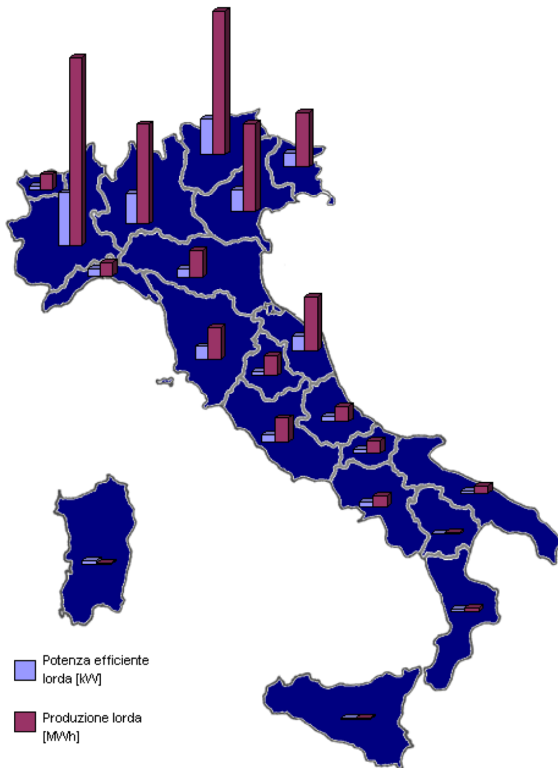
Figura 4.38: Dislocazione regionale degli impianti di PG alimentati da fonti rinnovabili (Potenza efficiente lorda totale: 493 MW; Produzione lorda totale: 1.682 GWh) 14 .
